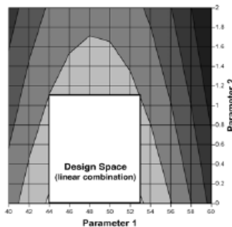
图1d: 制粒参数的设计空间，根据达到满意溶出度（即>80%）的参数范围的线性组合定义。
