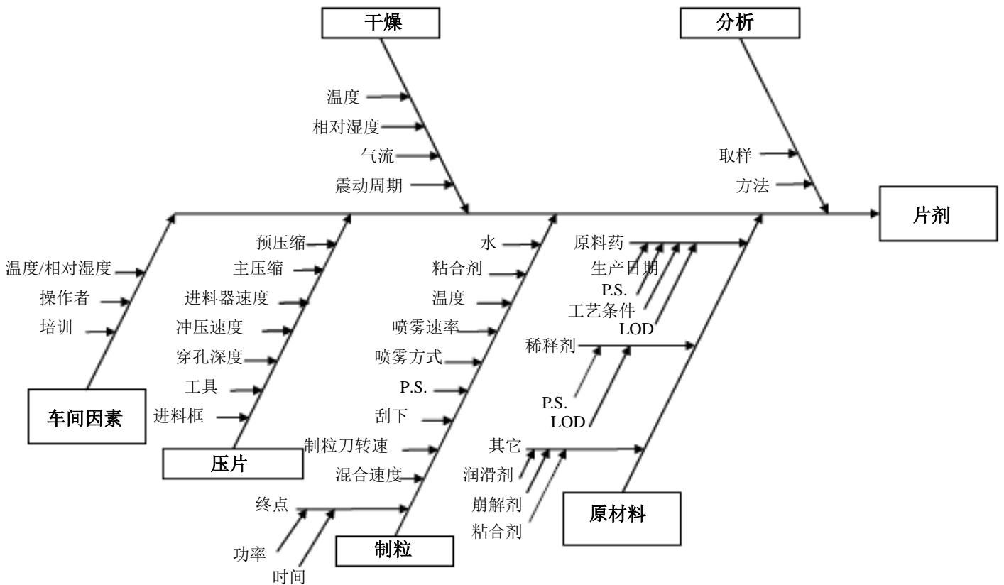
Ishikawa简图
