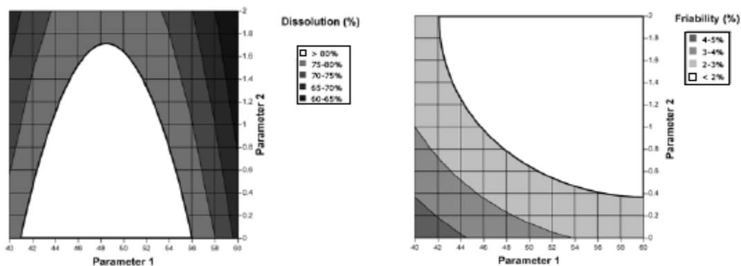
图 2a: 脆碎度作为参数 1 和 2 函数的指纹图。 图 2b: 溶出度作为参数 1 和 2 函数的指纹图。
